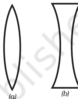
चित्र 15.22 (a) उत्तल लेंस तथा (b) अवतल लेंस
